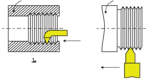
صورة (9): أقلام خراطة القلاووظ
