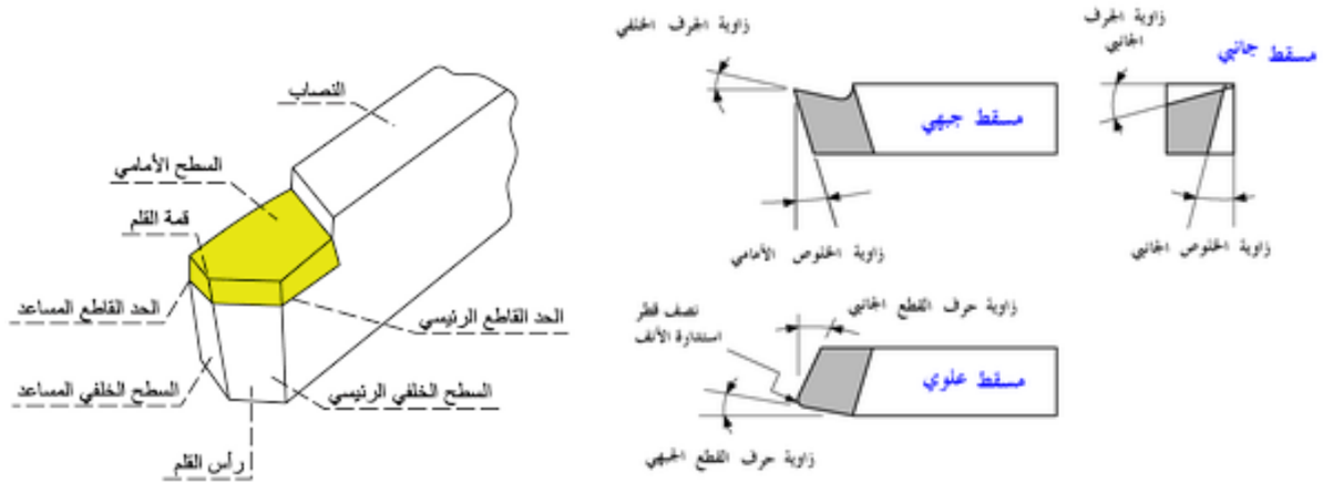
صورة (1): أجزاء قلم القطع و الزوايا.
