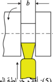
صورة (5): أقلام خراطة المجاري
